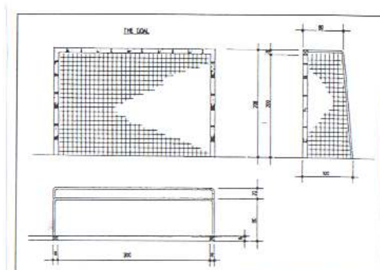
Skica 3: vrata 3 x 2 m za mali nogomet;
