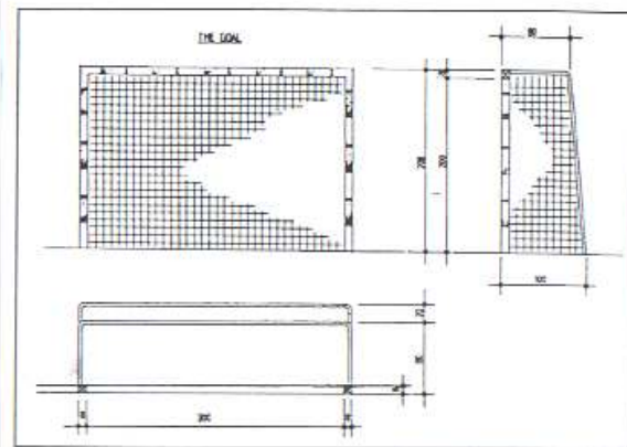
Skica 3: vrata 3 x 2 m za mali nogomet;
